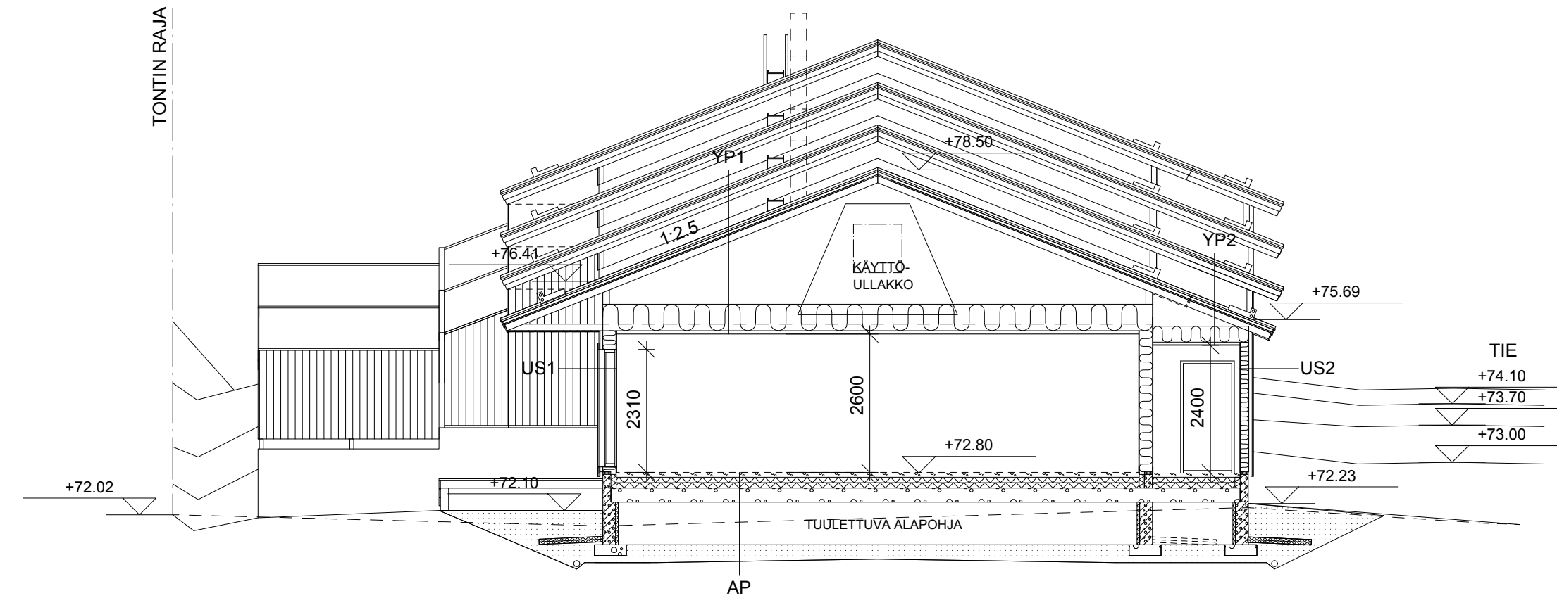
LEIKKAUS A-A
