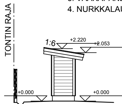
PÄÄTY ITÄÄN
