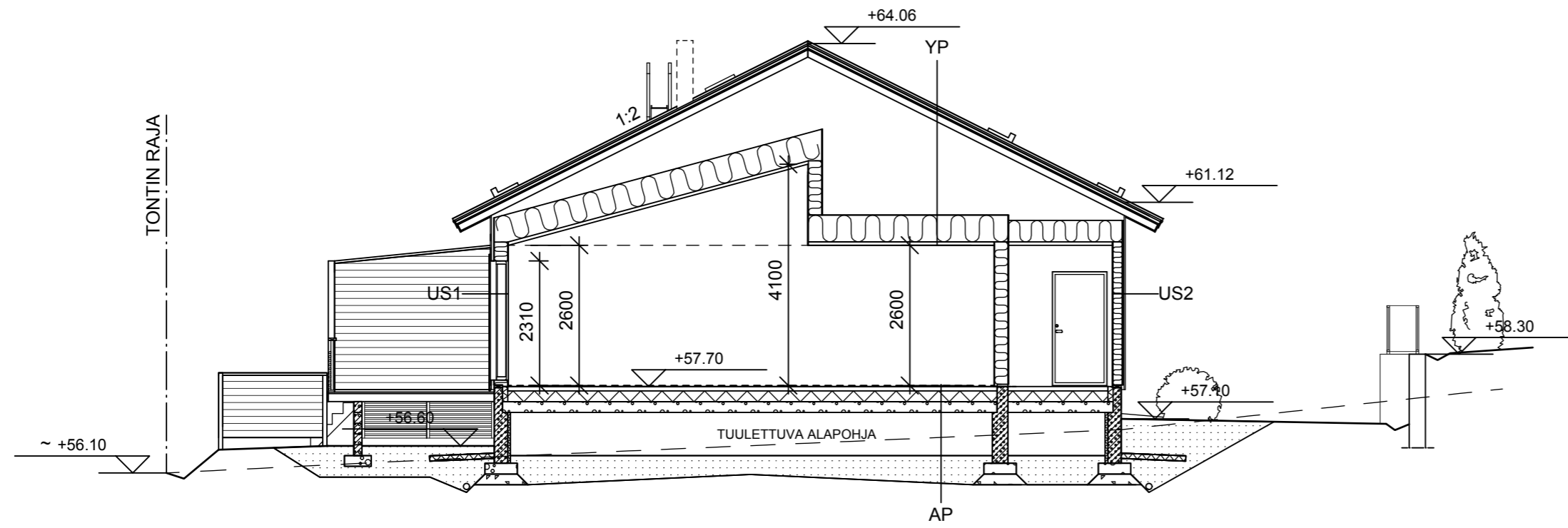
LEIKKAUS A-A
